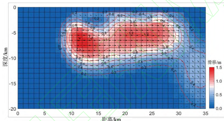
图 3 基于 InSAR 数据反演的同震滑动分布模型
