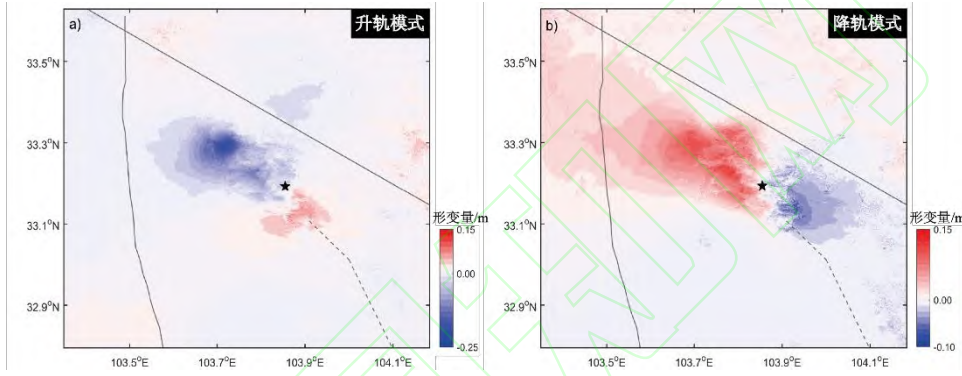
图2 九寨沟地震InSAR同震形变场
