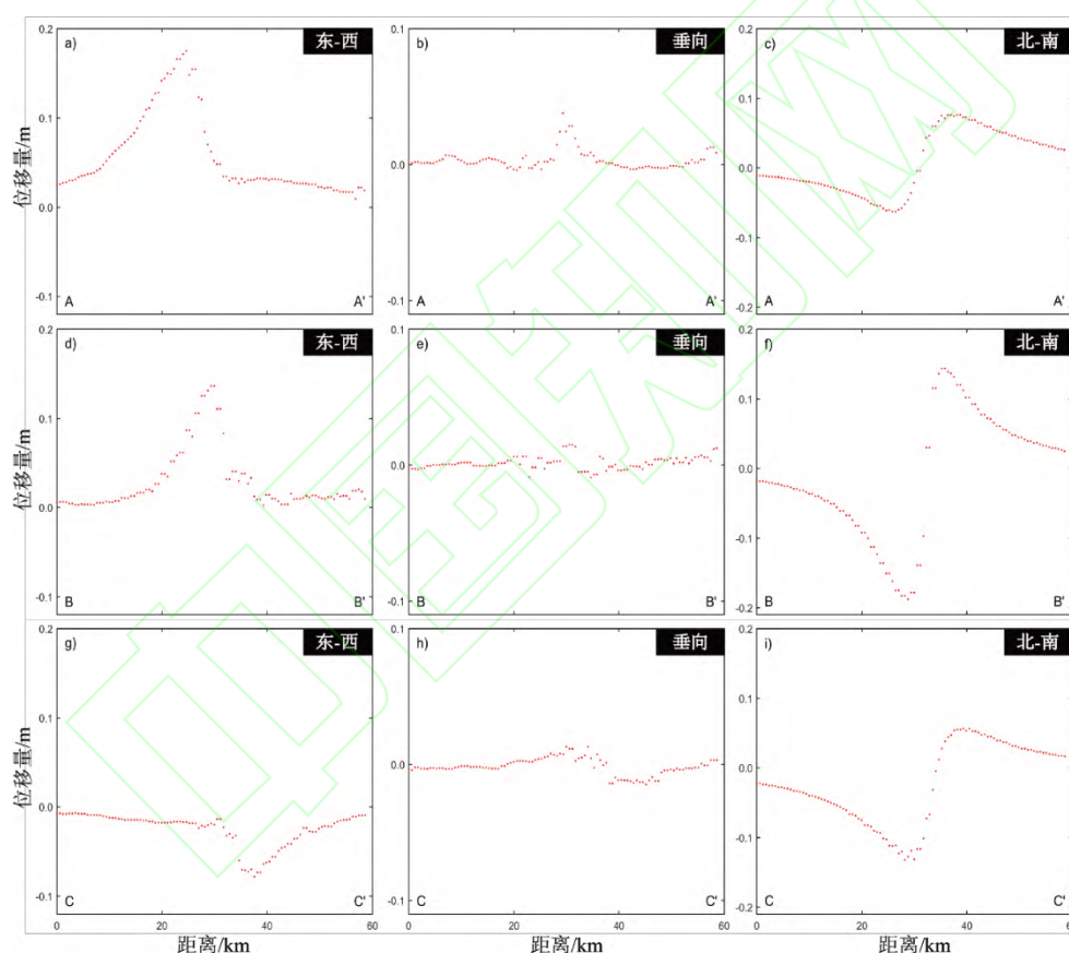
图 5 九寨沟地震三维形变剖面图
