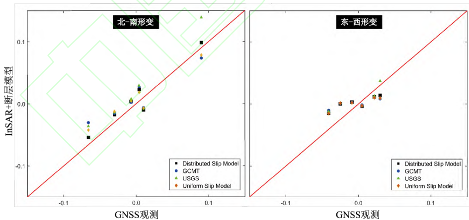
图 6 GPS 观测与解算结果一致性比较
