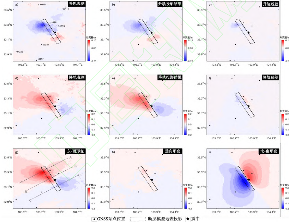
图 4 2017 年九寨沟地震 InSAR 观测与三维形变解算结果
