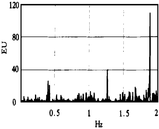
图 8 位移、水位频响函数曲线
