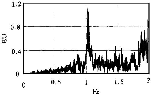
图 12 温度变化速度功率谱
