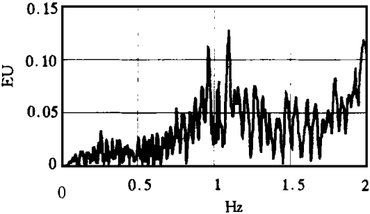
图 11 水位变化速度功率谱
