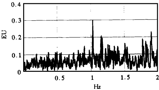
图 5 位移功率谱曲线 Fig. 5 Power Spectrum of Deformation
